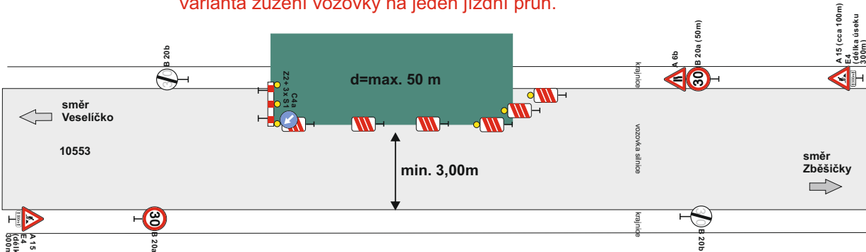
Schéma pracovního místa na silnici III/10553 v obci. Varianta zúžení vozovky na jeden jízdní pruh.
