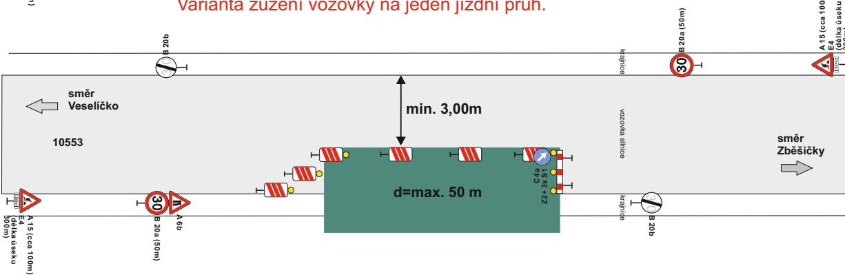
Schéma pracovního místa na silnici III/10553 v obci. Varianta zúžení vozovky na jeden jízdní pruh.
