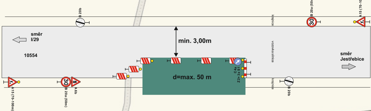
Schéma pracovního místa na silnici III/10554 v obci. Varianta zúžení vozovky na jeden jízdní pruh.
