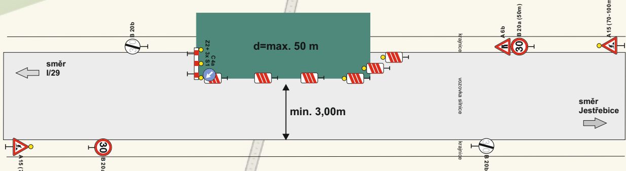
Schéma pracovního místa na silnici III/10554 v obci. Varianta zúžení vozovky na jeden jízdní pruh.
