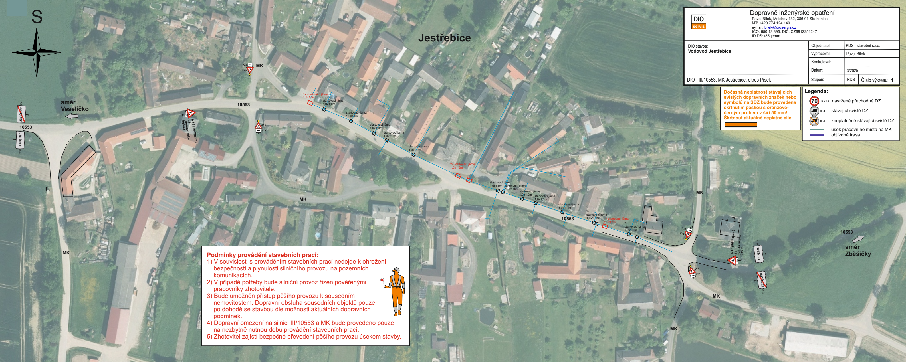
Schéma pracovního místa na silnici III/10553 v obci. Varianta zúžení vozovky na jeden jízdní pruh.
